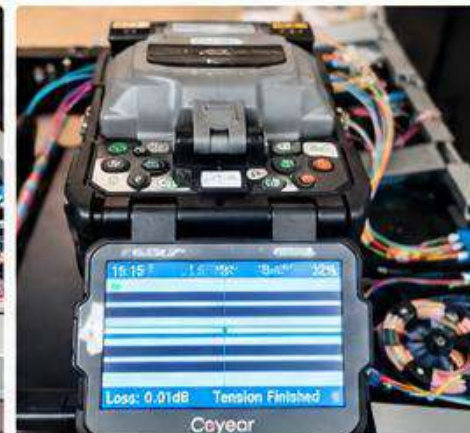
Proceso de fusión de fibra óptica.
