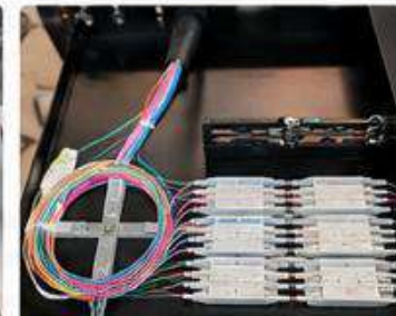
Identificación y organización de empalmes.
