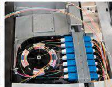
Gestión y acomodo de fibras.
